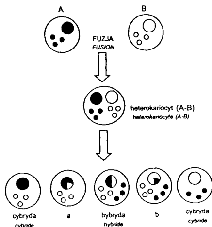
Ryc. 3. Fuzja dwóch genetycznie różnych protoplastów; a i b: hybrydy asymetryczne [wg 42, zmodyfikowane].
