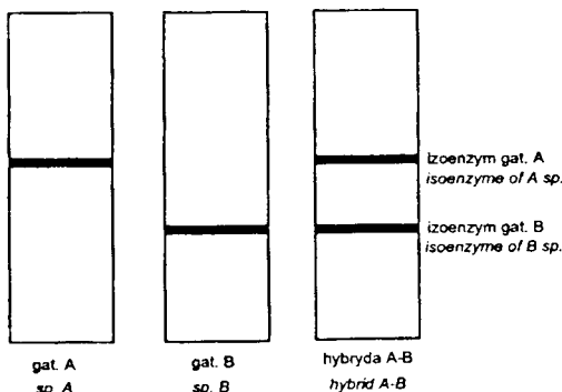
Ryc. 4. Wykrywanie form hybrydowych poprzez rozdział elektroforetyczny izoenzymów.
